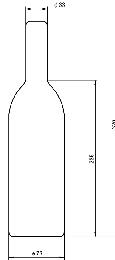
图 C.1 测试酒瓶尺寸示意图
